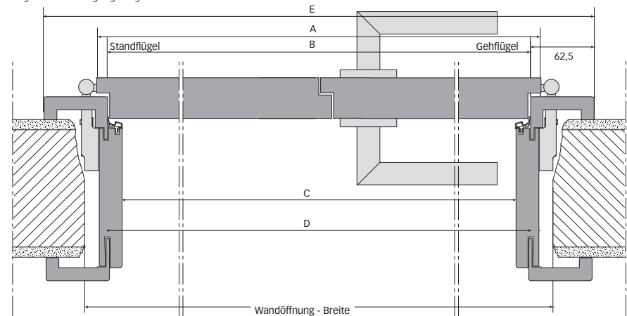
2-flg. Einzelanfertigungszarge
