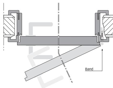
DIN rechts
